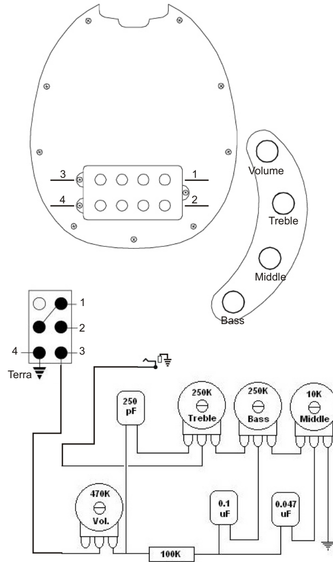
Esquema utilizando 1 MM4 ou Mm5 Alnico
