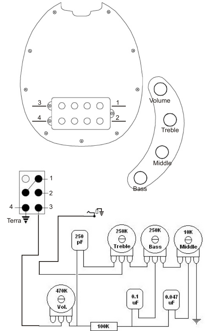
Esquema utilizando 1 MM4 ou Mm5 Alnico
